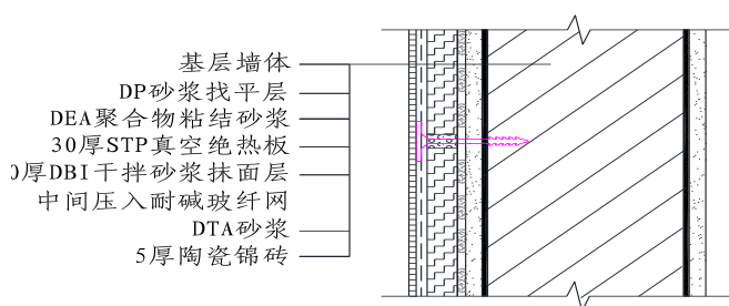
图一 外墙保温基本构造
