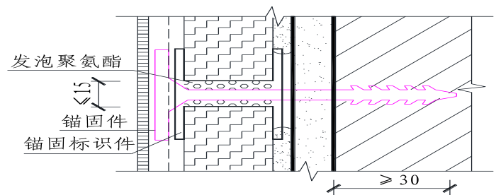
图二 锚固及板缝处理示意图
